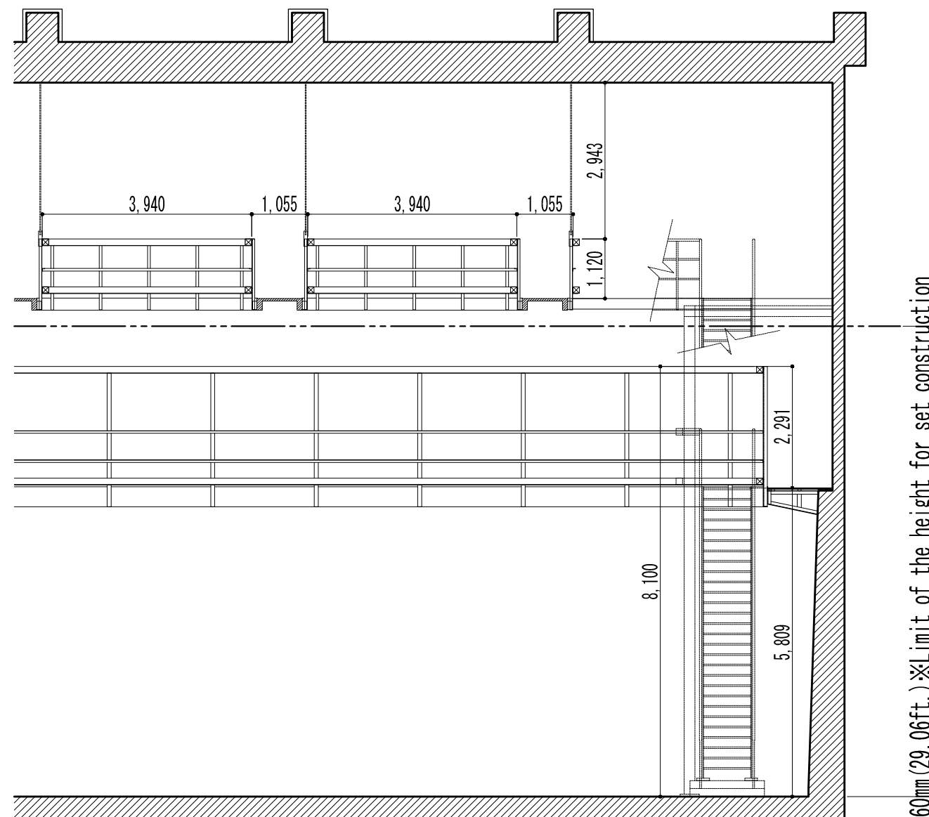
X-X' 断面図
